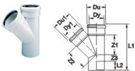
Тройник 67°
