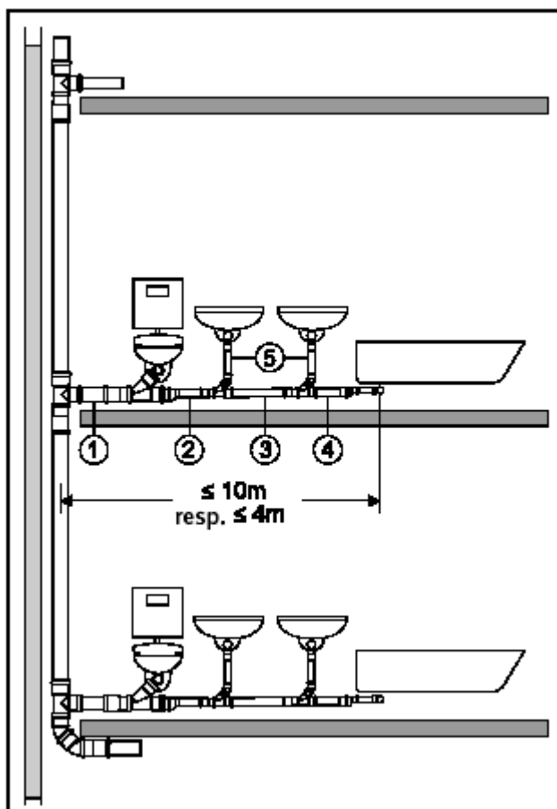
Рис. 11: Сборно-соединительный трубопровод
