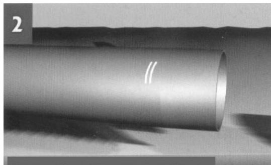
2 Нанесение линии ограничения на гладком конце трубы
