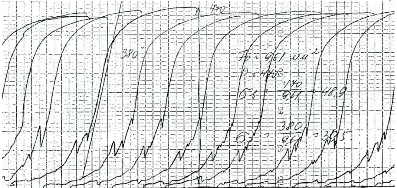
Рис. 3.3 Диаграмма растяжения образца из ВЧШГ при заводских испытаниях ОАО «Липецкий металлургический завод «Свободный Сокол»
