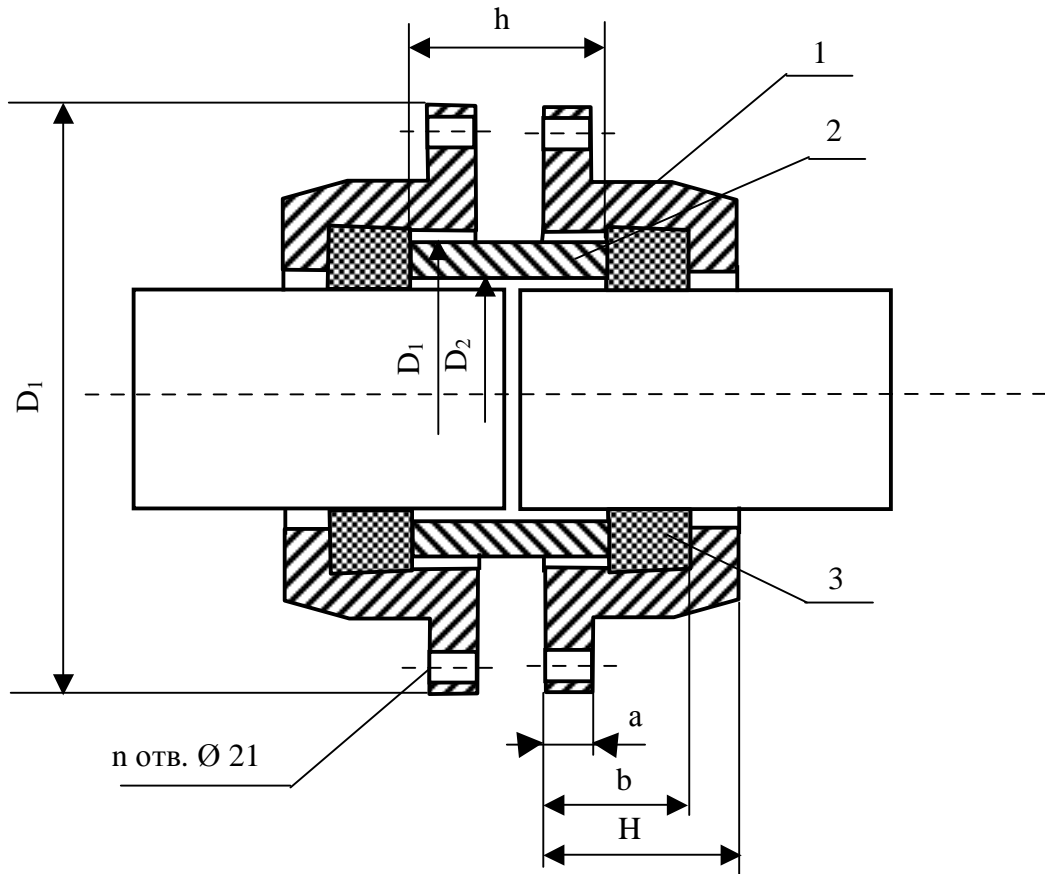
Рис. А.11 Муфтовое соединение (тип 1) 1 – муфта, 2 – втулка, 3 – резиновое кольцо
