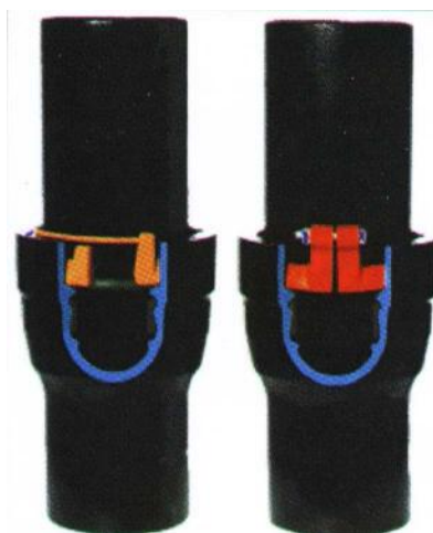
Рис. 5. 9 Раструбные соединения типа «ВРС»
