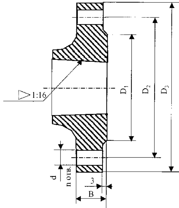
Рис. А.10 Схема фланца из высокопрочного чугуна (тип Б)
