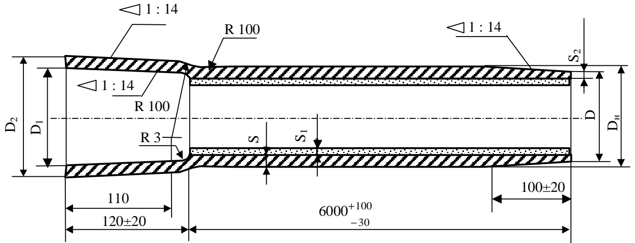
Рис. А.4 Схема трубы под нахлестное сварное соединение
