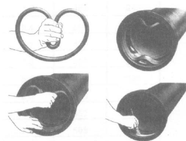
Рис. 5. 3 Схема укладки уплотнительного резинового кольца
