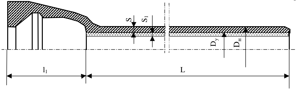
Рис. А.3 Схема трубы раструбной под соединение «Универсал»
