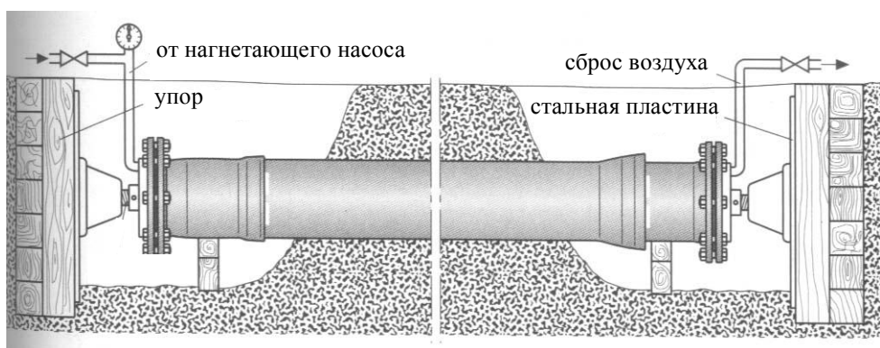
Рис. 5. 11 Подготовка трубопровода к гидроиспытанию
