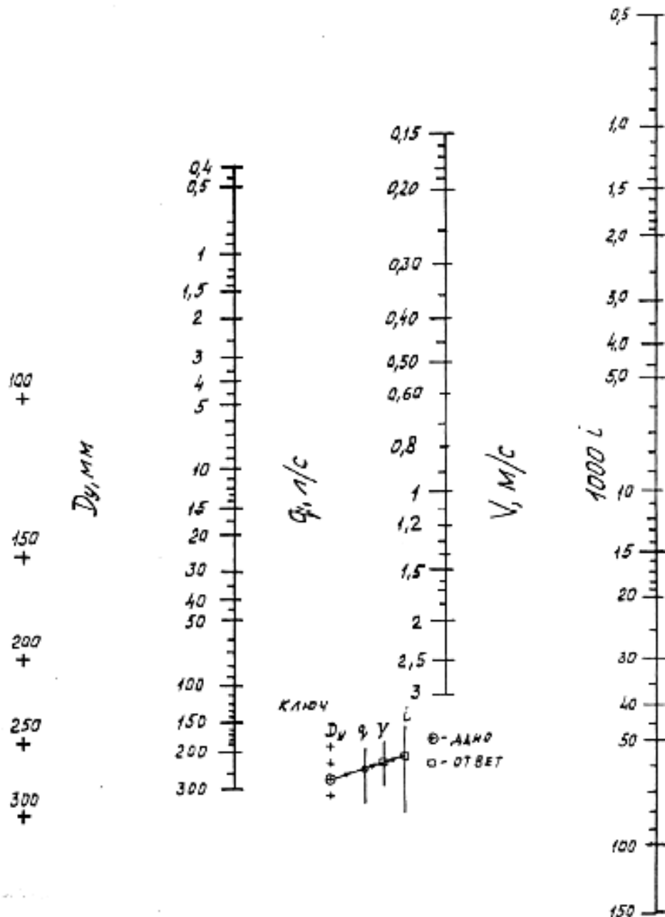
Рис. В.1 Номограмма расчета труб с внутренним цементно-песчаным покрытием производства ОАО «Липецкий металлургический завод «Свободный Сокол»
