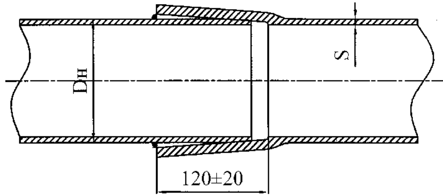
Рис. А.5 Схема сварного нахлестного соединения
