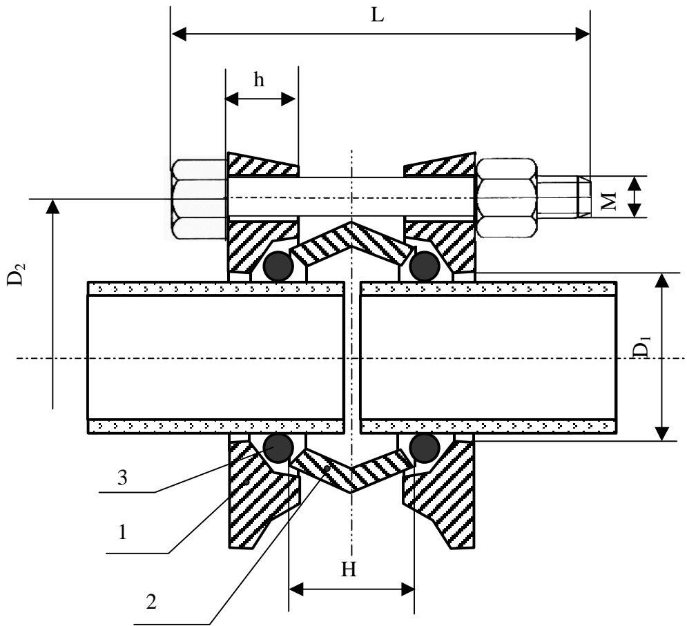
Рис. А.12 Муфтовое соединение (тип 2) 1 – фланец, 2 – втулка, 3 – резиновое кольцо
