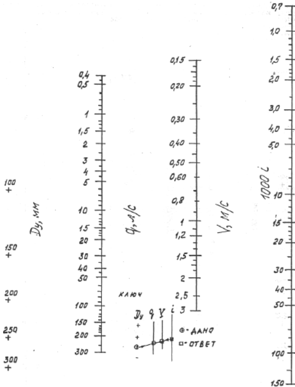
Рис. В.2 Номограмма расчета труб без внутреннего цементно-песчаного покрытием производства ОАО «Липецкий металлургический завод «Свободный Сокол»
