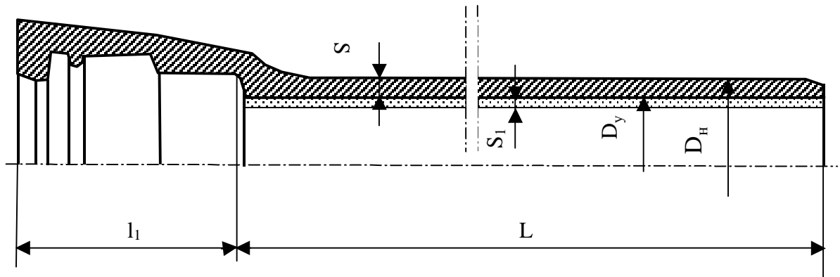
Рис. А.1 Схема трубы раструбной под соединение «Тайтон»
