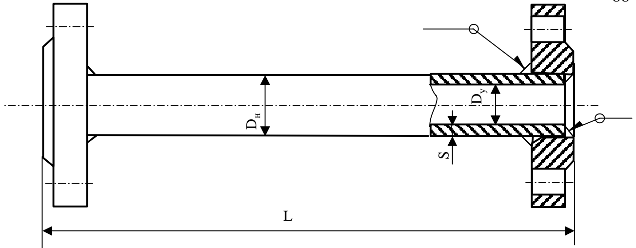
Рис. А.7 Схема трубы с приваренными фланцами (тип А)
