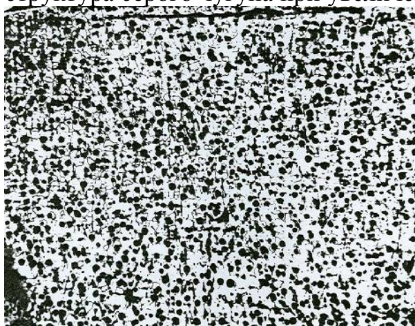
Рис. 3.2 Примерная структура чугуна с шаровидным графитом при увеличении шлифа в 100 раз
