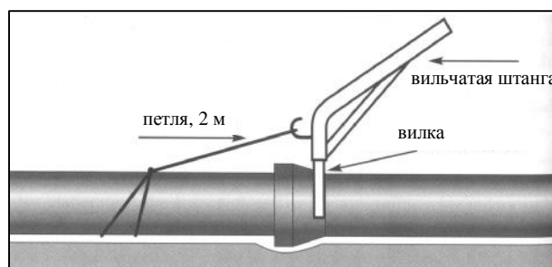
б) при помощи петли и вилчатой штанги (для Ду 100-150)
