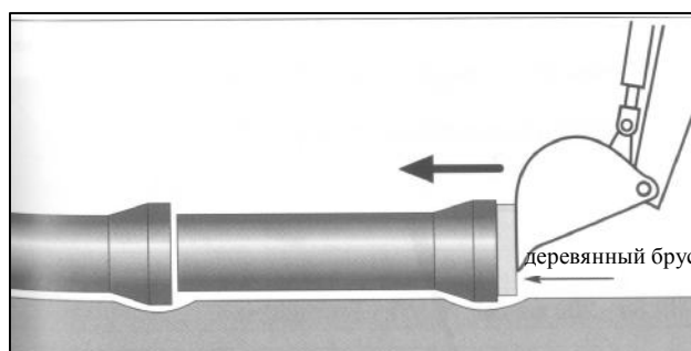
г) при помощи экскаватора и деревянного бруса (для Ду 100-300)
