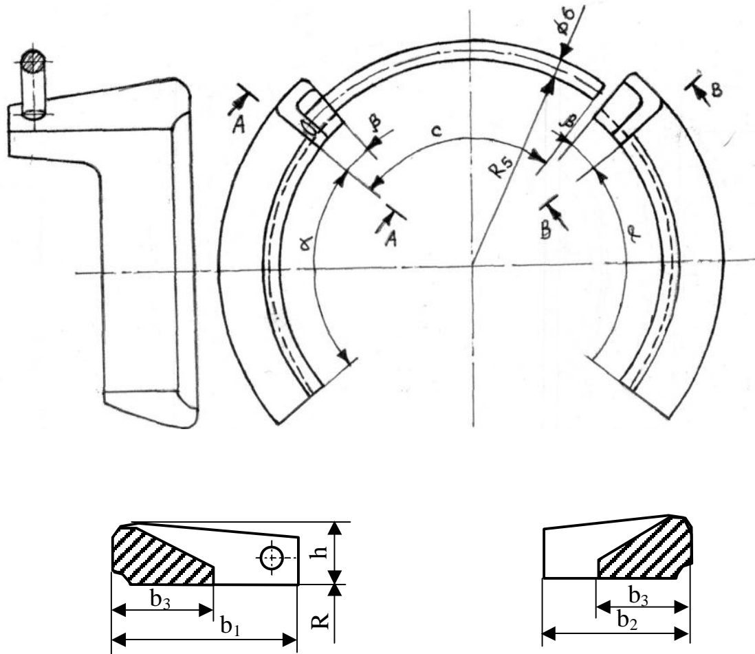
Рис. А.6 Схема стопоров из ВЧШГ (под соединение «ВРС»)
