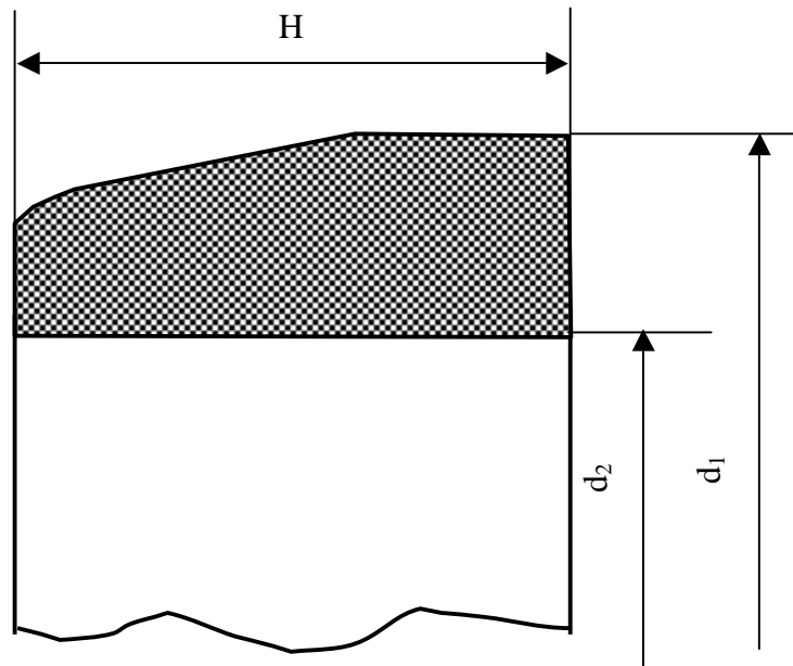
Рис. А.16 Уплотнительное резиновое кольцо для муфтового соединения (тип 1)
