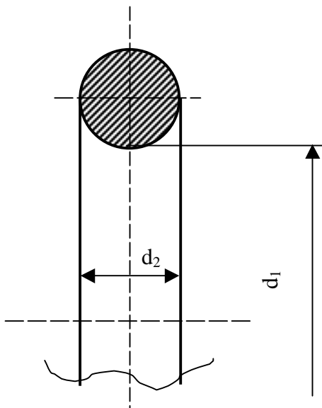
Рис. А.17 Уплотнительное резиновое кольцо для муфтового соединения (тип 2)
