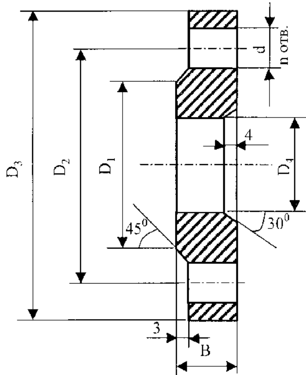
Рис. А.9 Схема фланца из высокопрочного чугуна (тип А)
