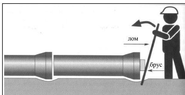
а) при помощи лома и деревянного бруса (для Ду 100)
