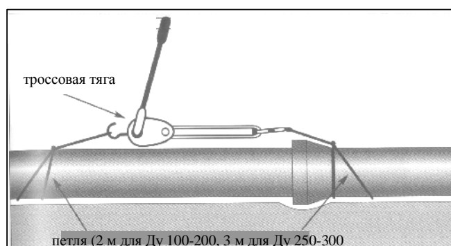
в) при помощи петли и тросовой тяги (для Ду 100-300)
