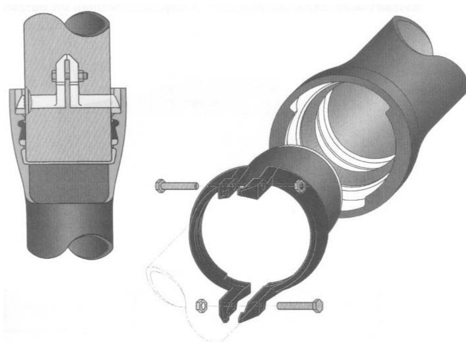
Рис. 5. 4 Специальное приспособление, заменяющее наплавленный валик
