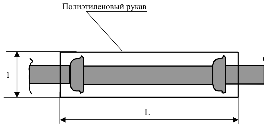
Рис. 4.1 Схема нанесения полиэтиленового рукава на трубу
