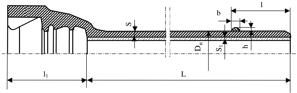
Рис. А.2 Схема трубы раструбной под соединение «ВРС»
