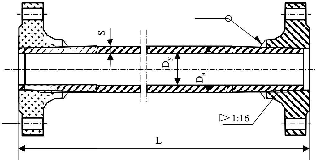
Рис. А.8 Схема трубы с приваренными фланцами (тип Б)
