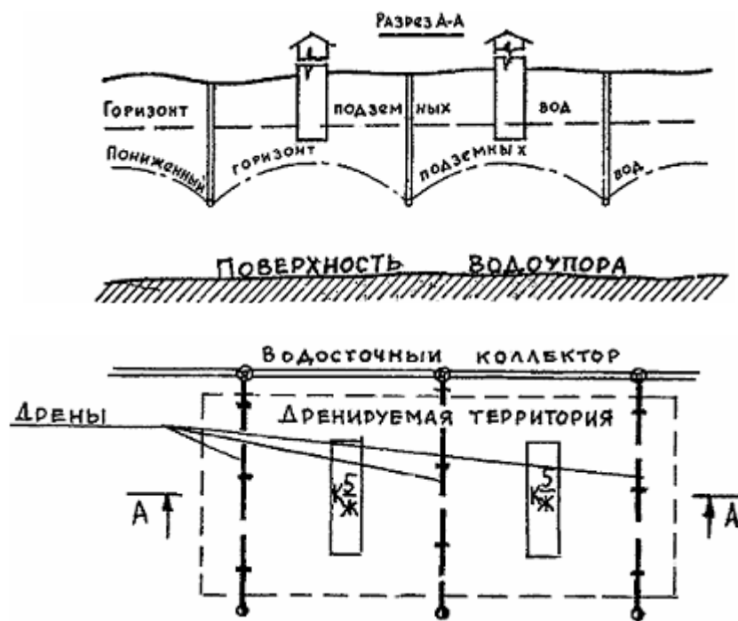
Рис.7. Схема систематического дренажа
