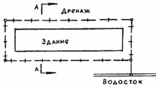
Рис.8. Схема кольцевого дренажа
