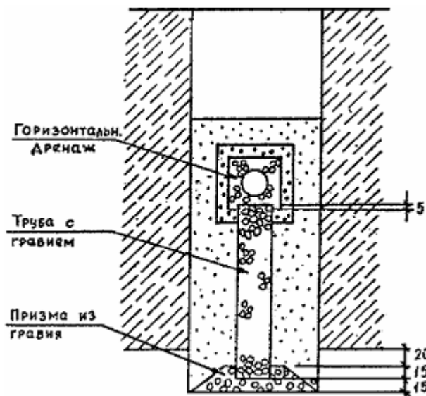
Рис.5. Комбинированный дренаж с вертикальным самоизливающимся колодцем
