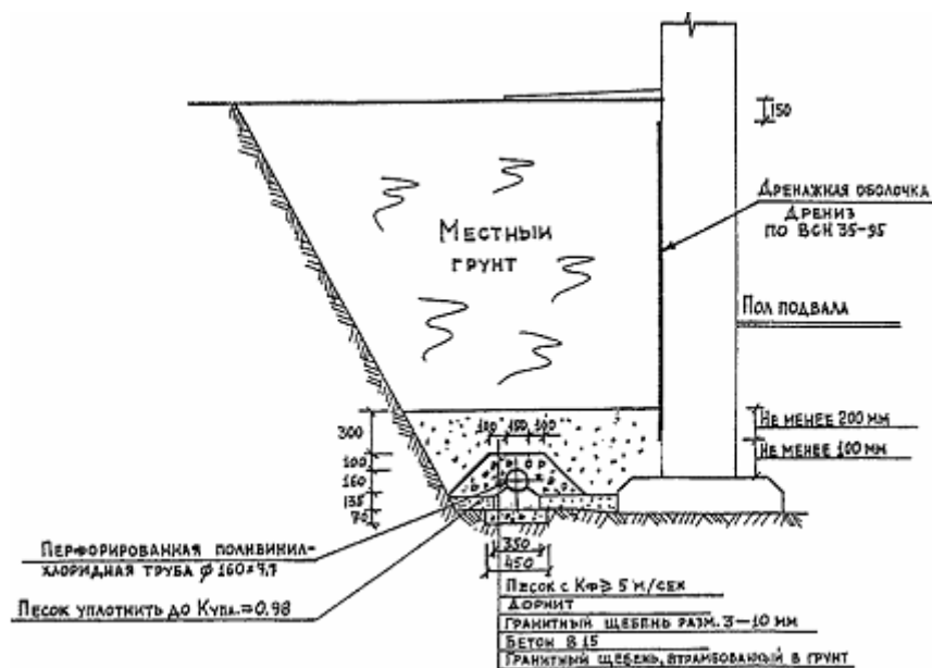
Рис.14. Пристенный дренаж с применением поливинилхлоридных труб
