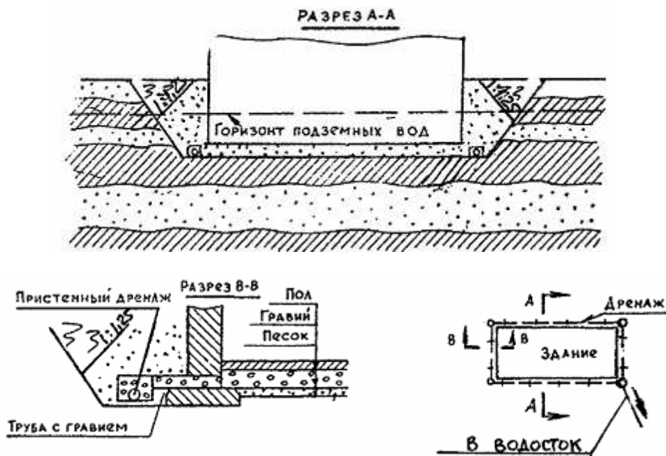
Рис.9. Схема пластикового дренажа
