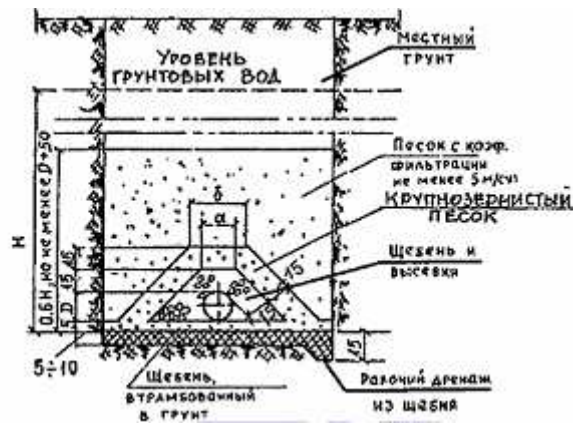
Рис.1. Дренаж совершенного типа
