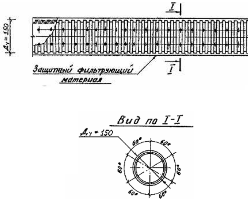
Рис.13. Труба гофрированная из полиэтилена низкого давления с водоприёмными отверстиями заводского изготовления
