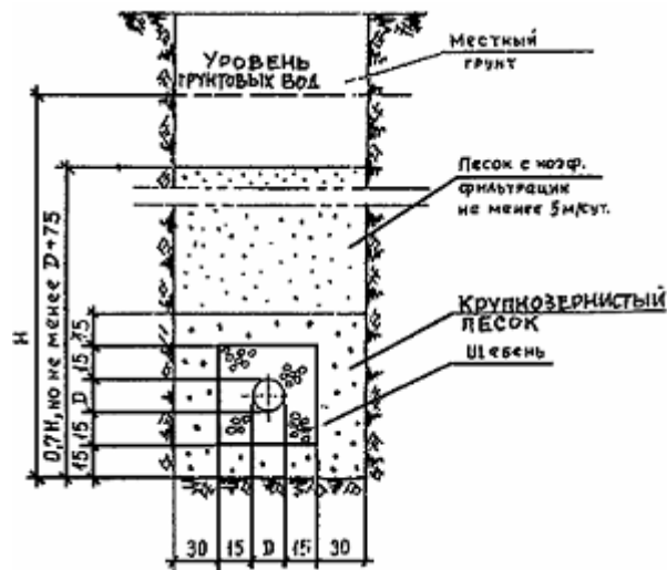
Рис.2. Дренаж несовершенного типа
