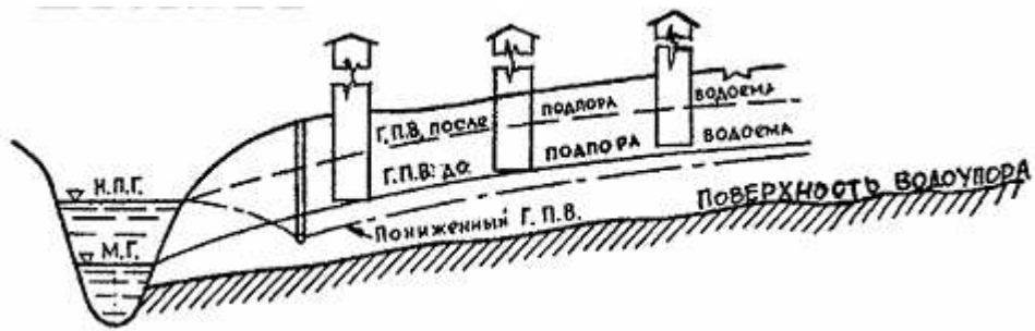
Рис.6. Схема берегового дренажа
