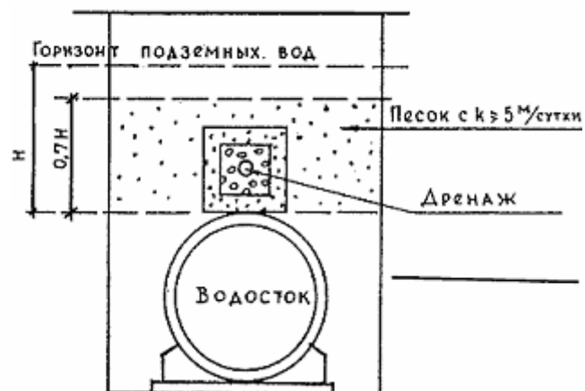
Рис.10. Схема прокладки дренажа над водостоком
